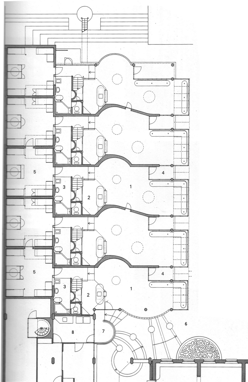
Aldo van Eyck, 1973-78, Hubertus / Mother's House, Amsterdam; zonas de juegos para niños Fuente: http://www.pieriniarchitettura.it/lab2015/?p=1076
