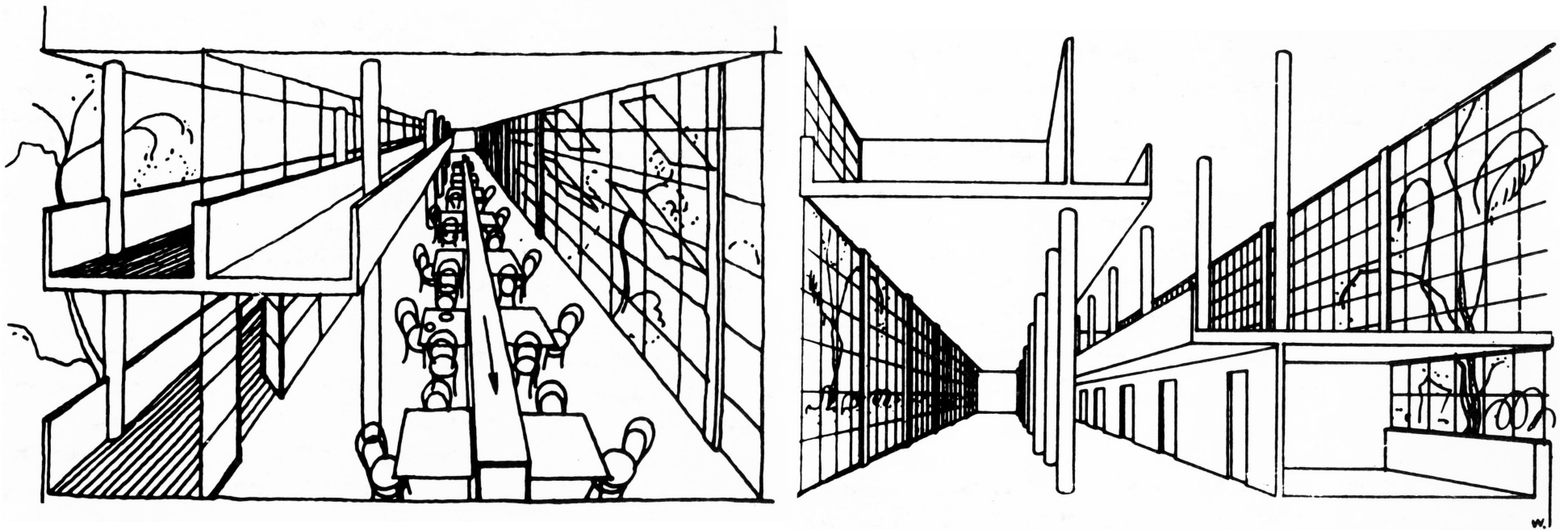
Barshch & Vladimirov, 1929, diseño de vivienda comunitaria en la URSS
